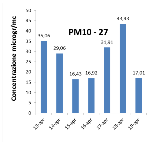
Figura 1: Concentrazioni medie giornaliere del PM 10
