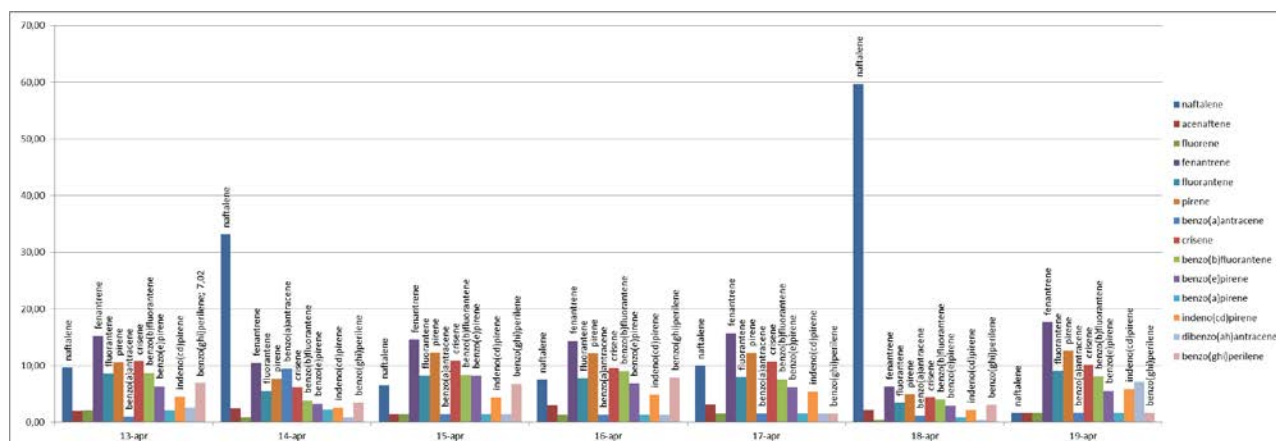
Figura 3: fingerprint delle miscele di IPA rilevate in ogni giorno del periodo studiato.
